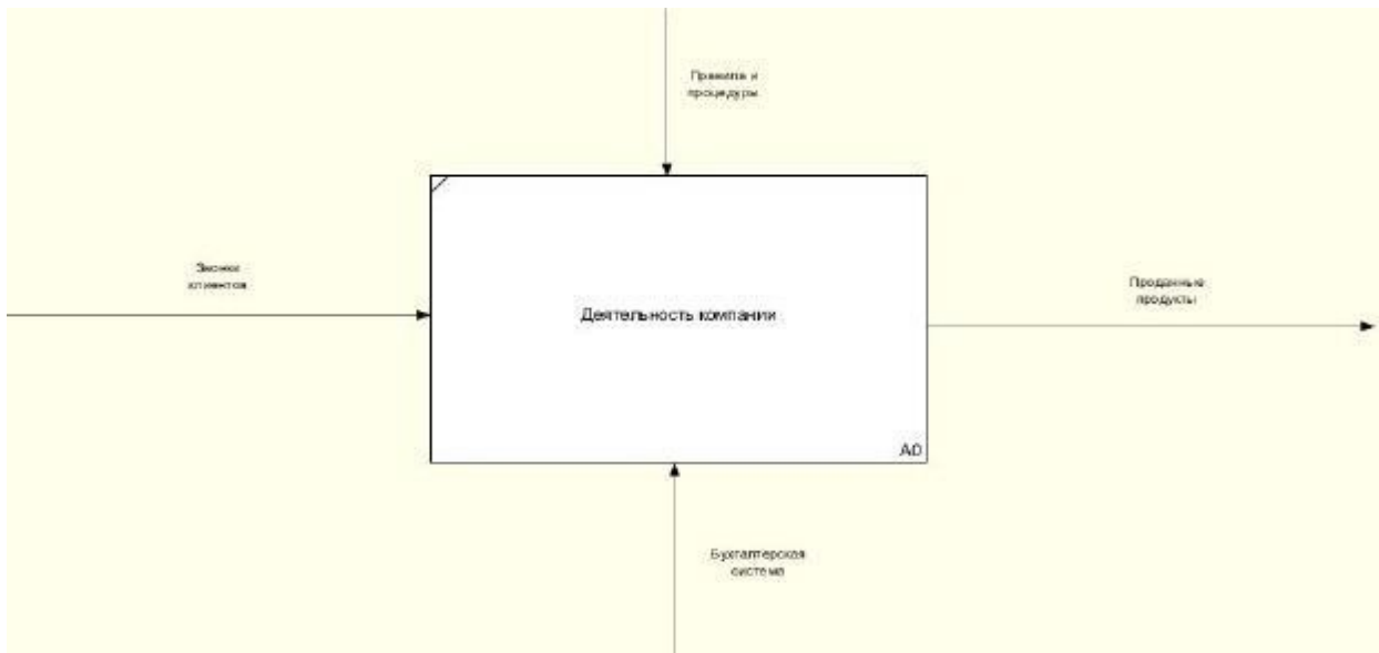
Рис. 2. Контекстная диаграмма
